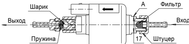
Рис. 5 – Топливный насос
