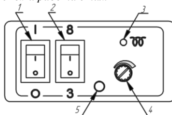
Рис. 4 – Лицевая панель пульта ПУ- 6
